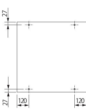
ボデー背面図 (遮光板を除く)
