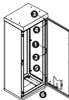
図5 ギャピンヒンジのはめ合わせ順序
