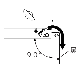
図 3 扉の外し方
