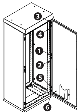
図 5 ギヤピンヒンジのはめ合わせ順序
