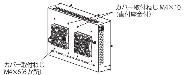
【OPCA-15R】 ドレンフィルタ取付方法
