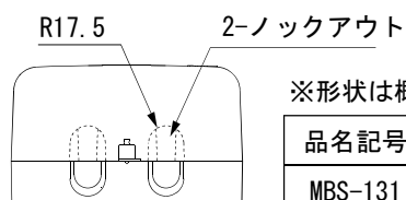
外形図
