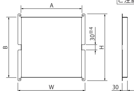
外形寸法
