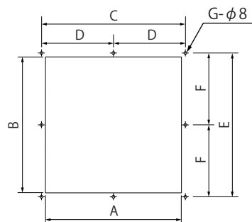
取付穴寸法
