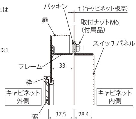
【取付時上部断面図】
