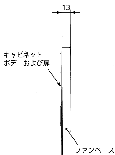
ファンベース取付時 BX-L80, BX-L120
