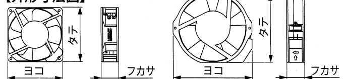
PF-121CL(-2)・PF-121L(-2)・ PF-185L(-2)
