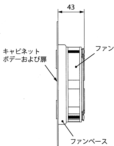
ファンベース+ファン取付時 BX-L80KL、BX-L120KL
