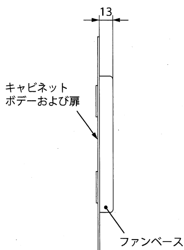
ファンベース取付時 BX-L80、BX-L120
