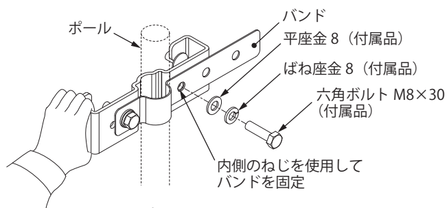
ボール径φ25～φ39の場合
